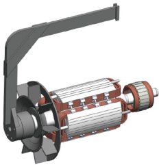
图11 用专用转子吊具吊装转子方法
