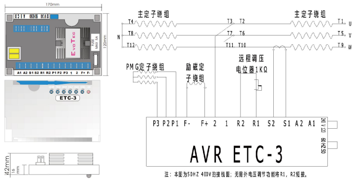
图6 ETC-3在400Vac系统接线图
