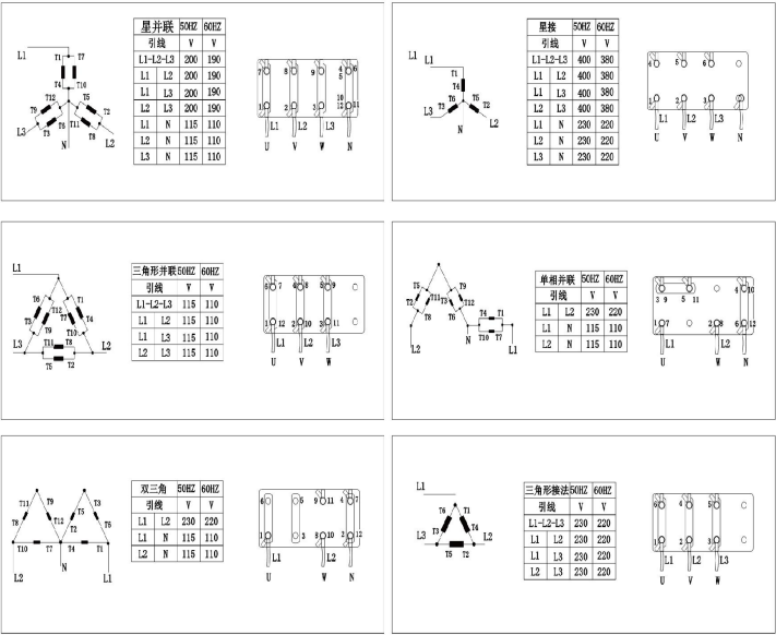
图10 50Hz/60Hz不同电压的接线方式图
