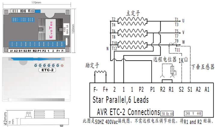
图5 ETC-2在400Vac系统接线图
