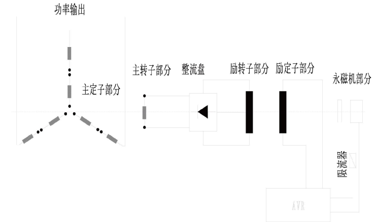
图2 PMG励磁电气原理图
