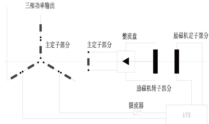
图1 自励电气原理图
