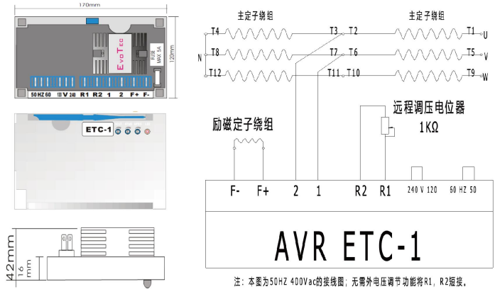
图4 ETC-1在400Vac系统接线图
