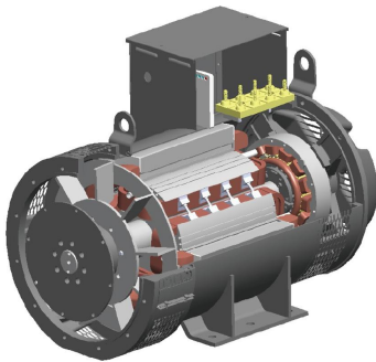
图3 发电机剖视图
